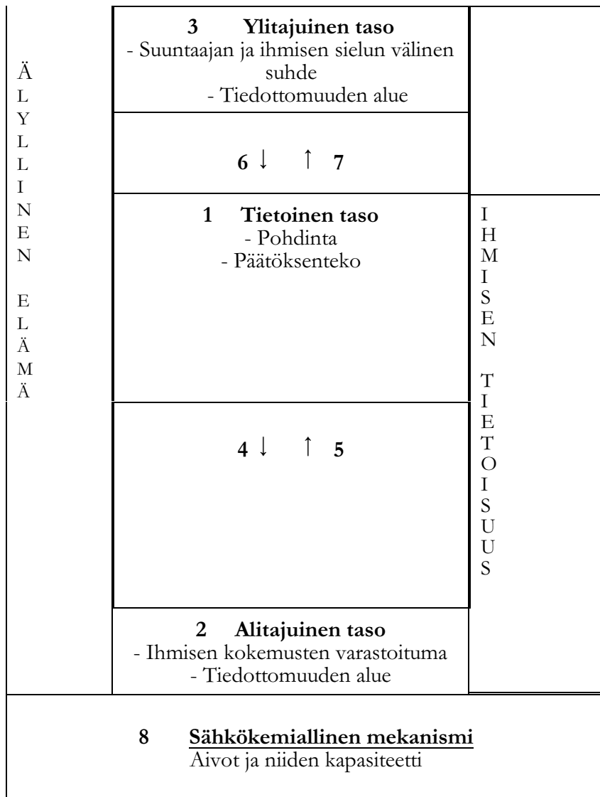
Kuva 1: Ihmismielen kaavio
